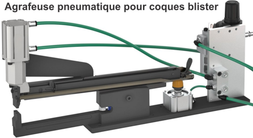
Agrafeuse pneumatique pour coques blister
